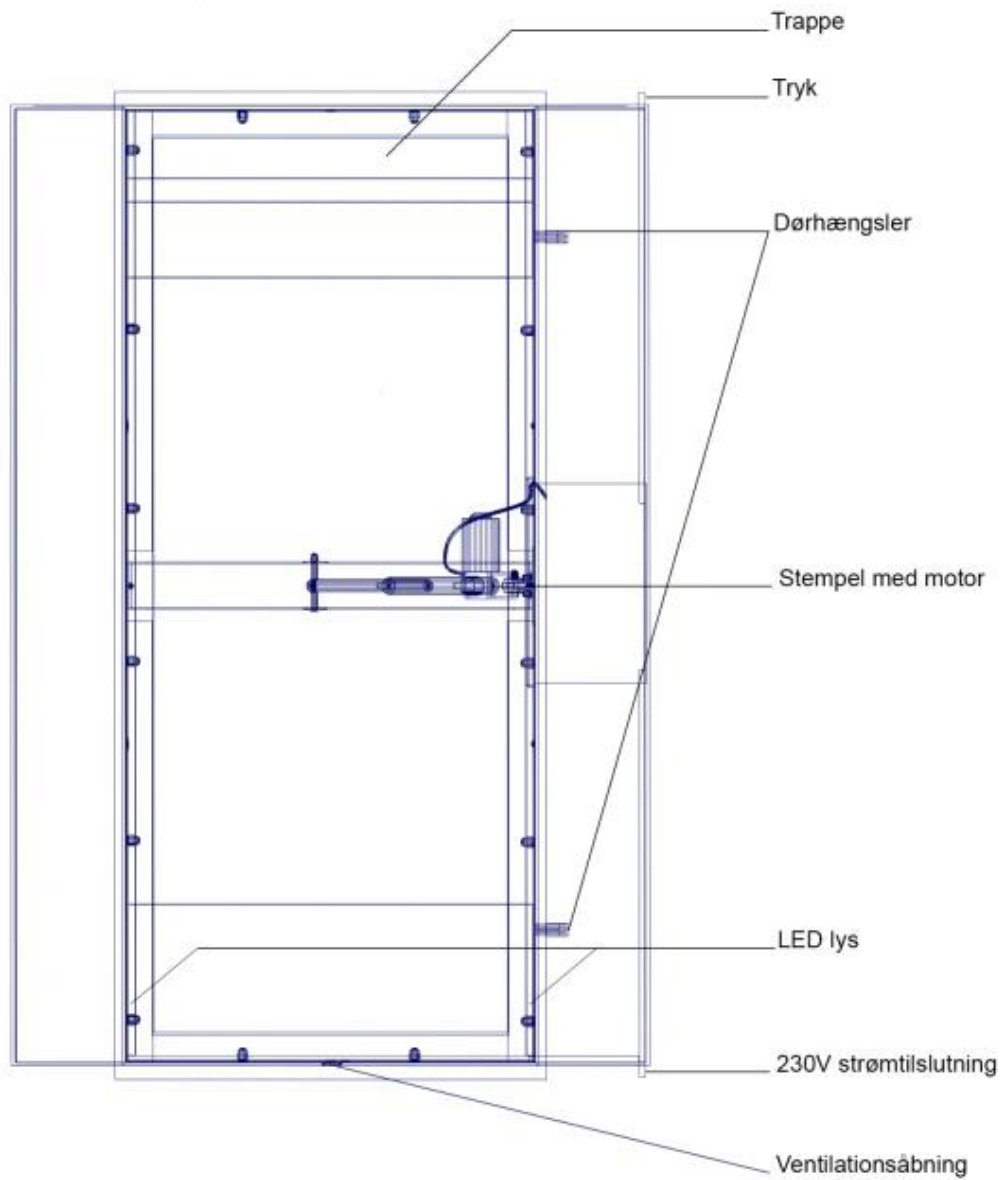
Konfiguration A
